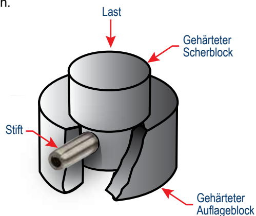
Scherversuch wurde in einer der ISO 8749 entsprechenden Vorrichtung durchgeführt
