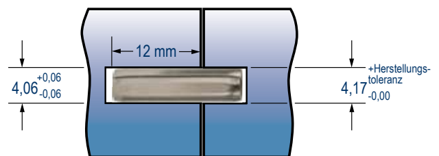
Empfohlenes Bohrungsmaß für Spießpassung bei CLDP 4 x 20 LBK
