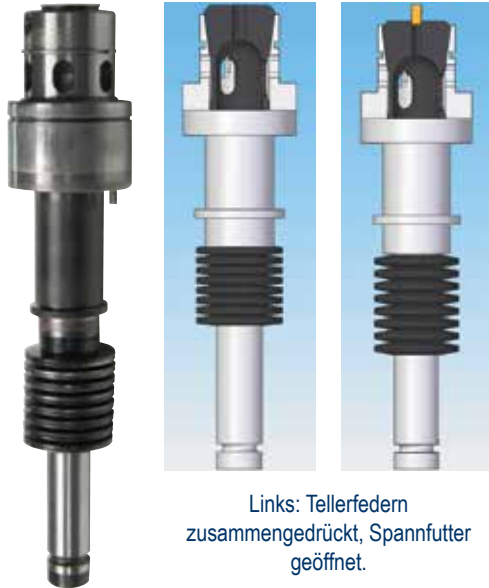
Rechts: Tellerfedern dekomprimiert, Spannfutter geschlossen, Werkstück umklammert.
